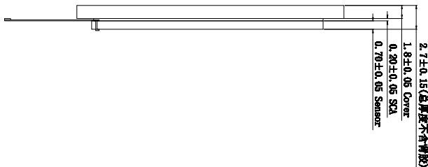
侧视图 横向10:1
