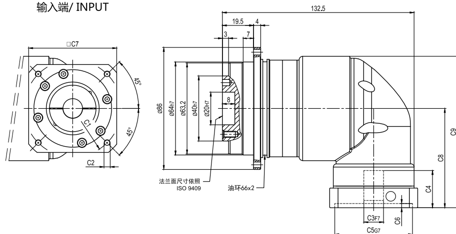
输入端/ INPUT
