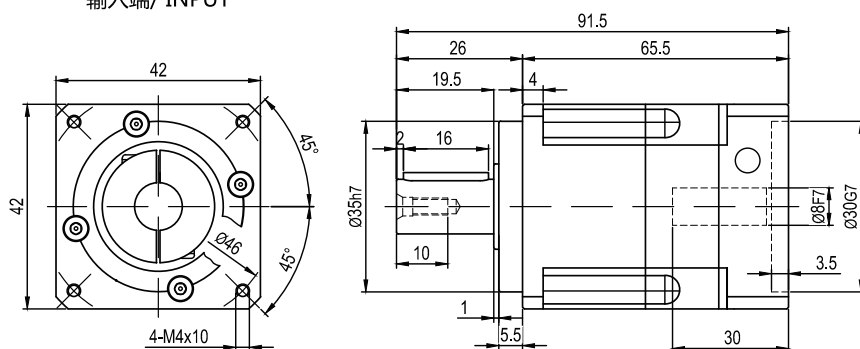
输入端/ INPUT
