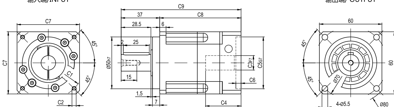
输出端/ OUTPUT
