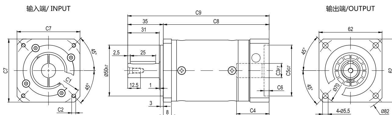
PGE60-L2
