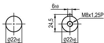
轴型式 S1
