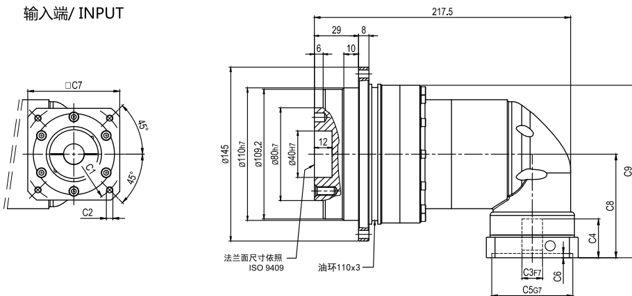
输入端/ INPUT
