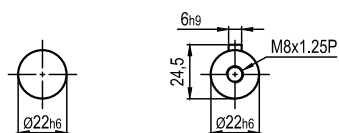
轴型式 S1
