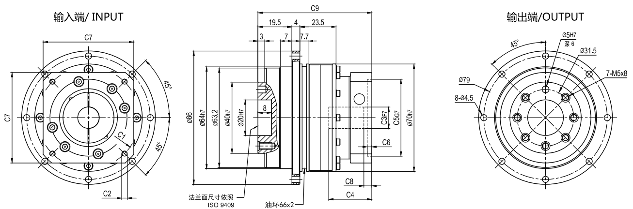
PGF60-L2
