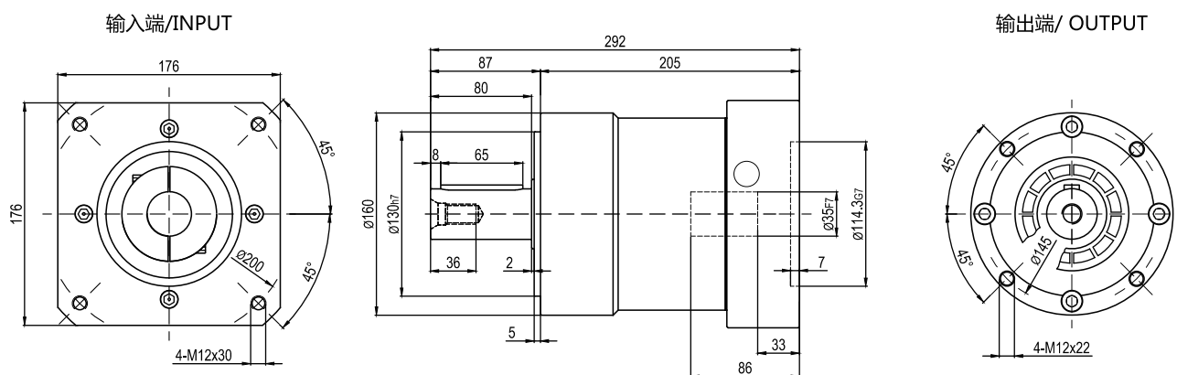
PGC160-L2
