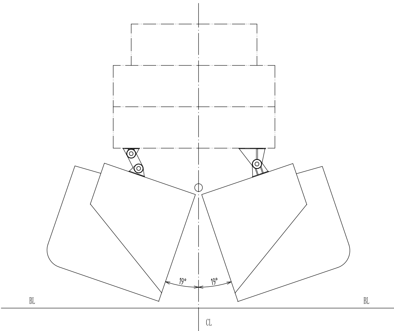
泥舱开体状态
