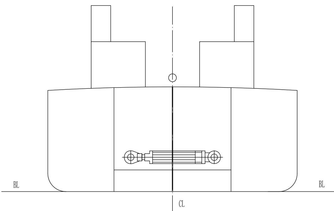
正浮状态
