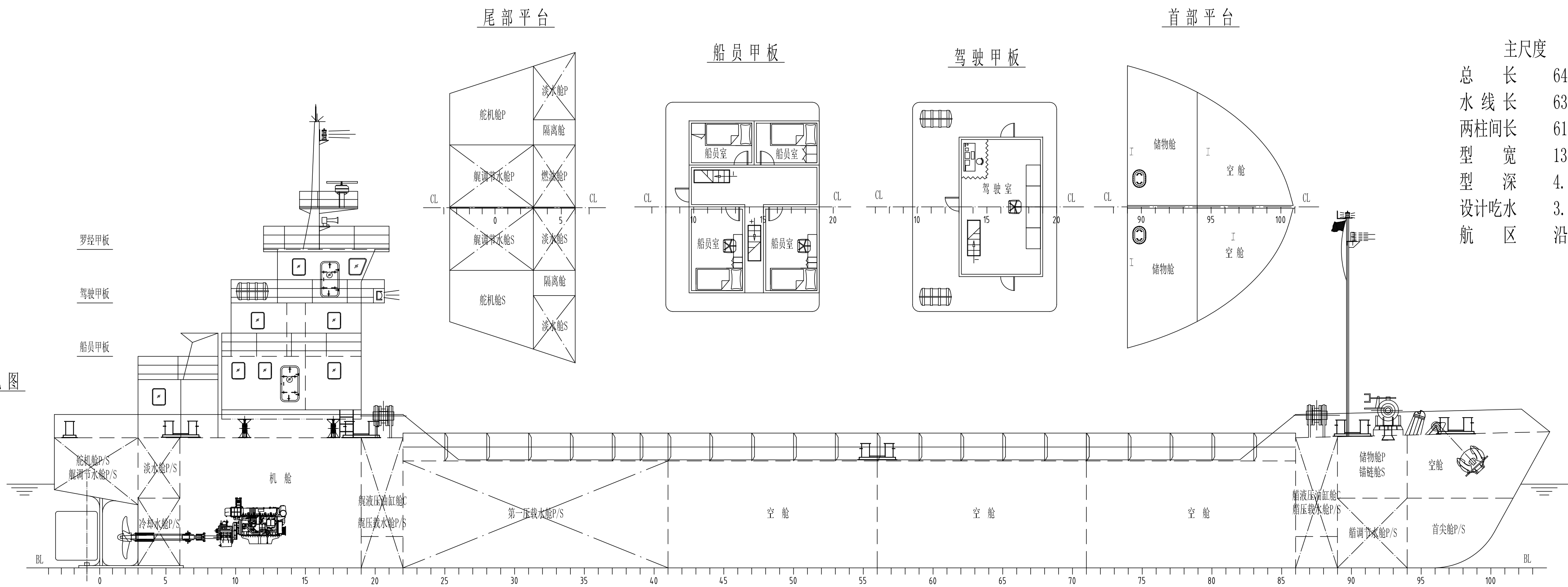
主甲板
