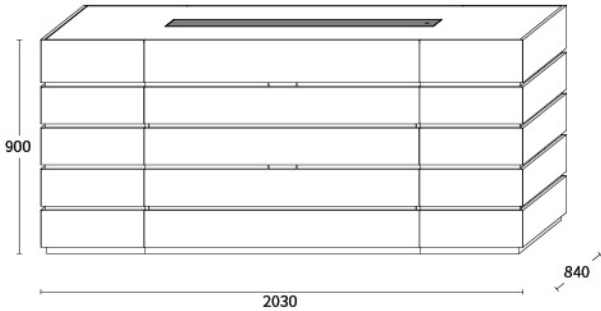
中岛台标准版-带摇表器功能模块
