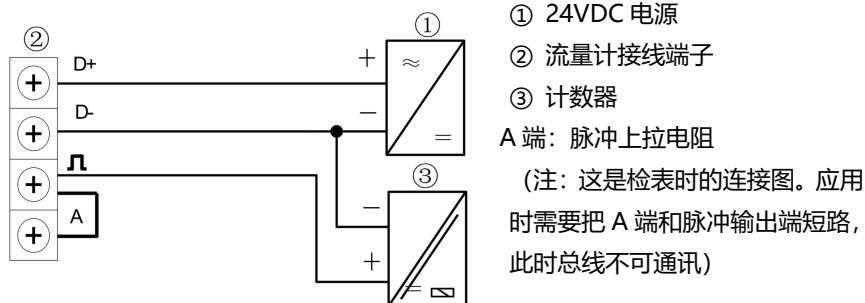
电气接线图
