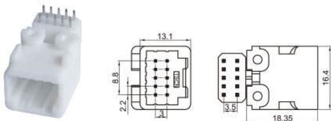
Type: TSTA10-10PM-PKB Material: PA66 Matching Terminal: TSPM0040 / TSPM0041
