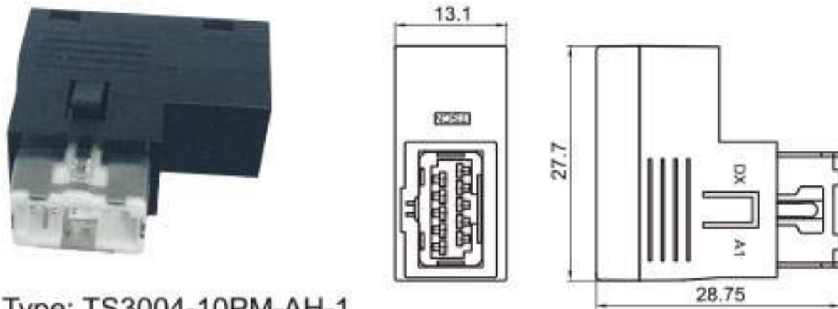
Type: TS3004-10PM-AH-1 Material: PA66 Matching Terminal: TSAM0031 / TSAM0032 / TS 长城 H6
