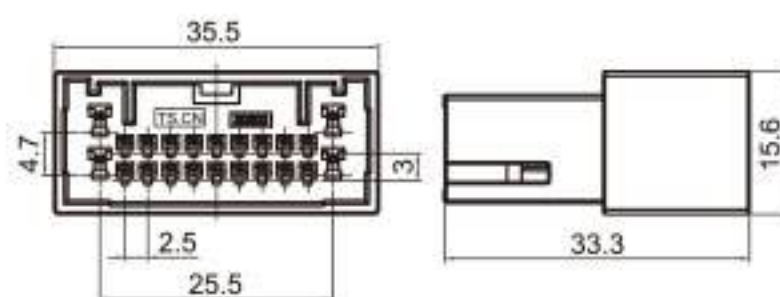
Type: TS30300-22P-11 Material: PBT Matching Terminal: TSZ619 / TSZ618
