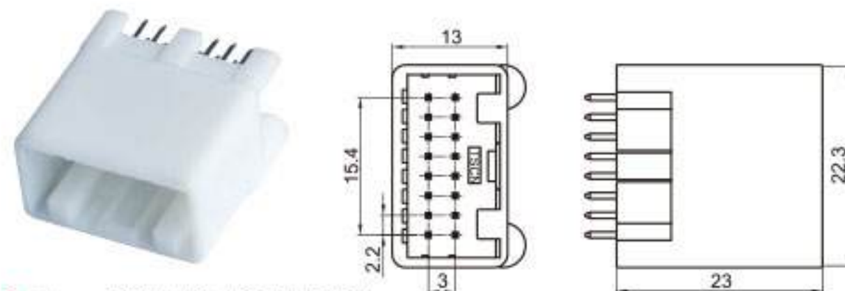
Type: TSTA16-16PM-PKS Material: PA66 Matching Terminal: TSPM0038
