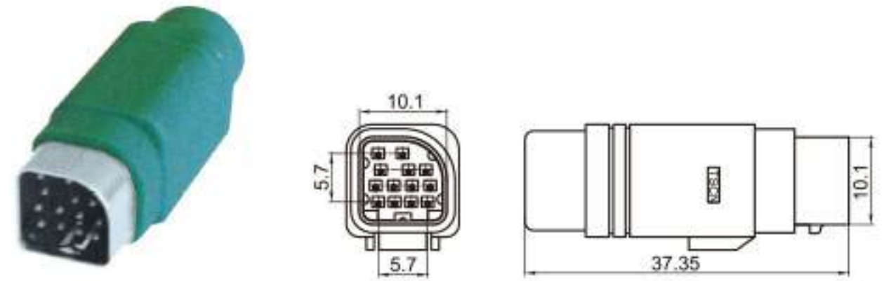
Type: TSALP13-13PM-AH Material: PA66 Matching Terminal: TSAM0016 / TSAM0015 / TS0079
