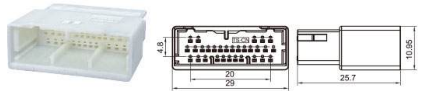
Type: TS30378-30P-11-1 Material: PA66 Matching Terminal: TSZ556
