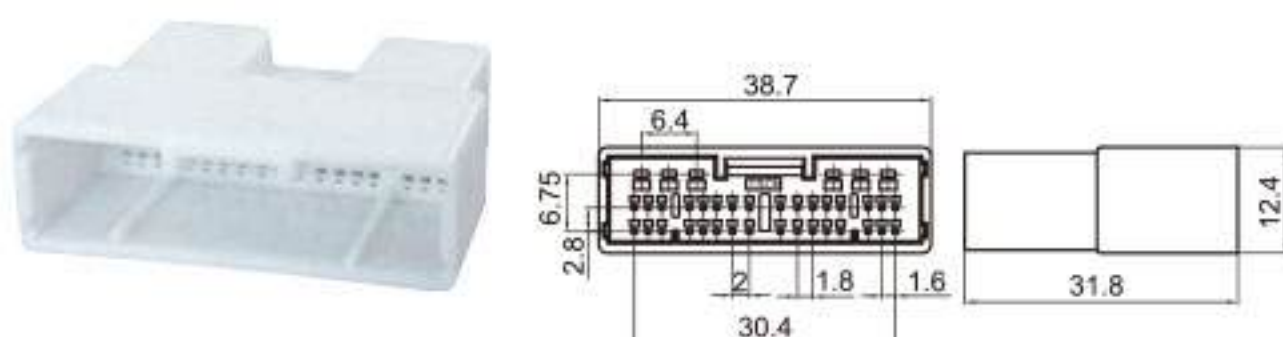
Type: TS30101-38P-11 Material: PA66 Matching Terminal: TSZ562 / TSZ556
