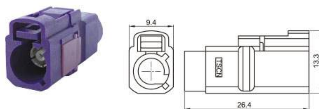
Type: TSVW20-01PF-AT-VT Material: PA66 GF30% Matching Terminal: TSTF0025 / TSTF0026
