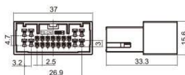
Type: TS30300-22P-11-1 Material: PBT Matching Terminal: TSZ619 / TSZ618
