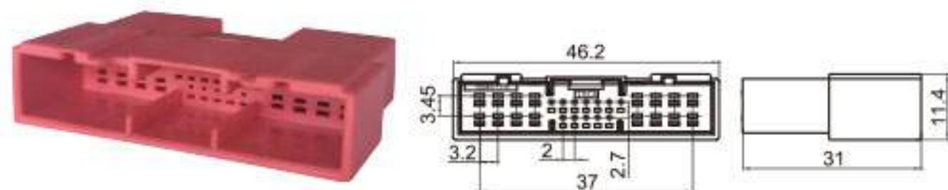
Type: TS30243-28P-11-5 Material: PBT Matching Terminal: TSZ040 / TSZ561A
