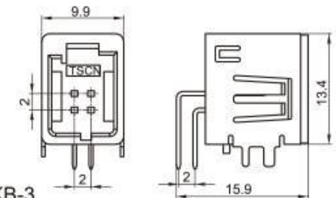
Type: TSMA04-04PM-PKB-3 Material: PPS Matching Terminal: TSPM0029-A / TSPM0031 / TSPM0032
