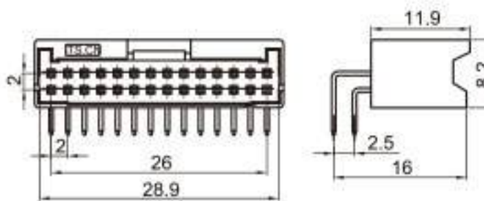
Type: TS30047-28PM-PKB(QRA3) Material: PA66 GF15% Matching Terminal: TSPM0143 / TSPM0144
