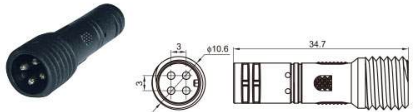
Type: TS 四芯防水公接头 Material: PVC Matching Terminal: TS1.5 圆头
