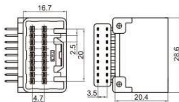
Type: TSMI18-18PM-PKB Material: PA66 Matching Terminal: TSPM0001 / TSPM0003
