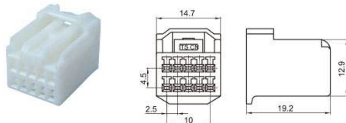
Type: TSTA10-10P-21 Material: PA66 Matching Terminal: TSH006
