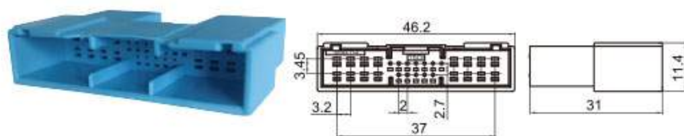
Type: TS30243-28P-11-4 Material: PBT Matching Terminal: TSZ040 / TSZ561A
