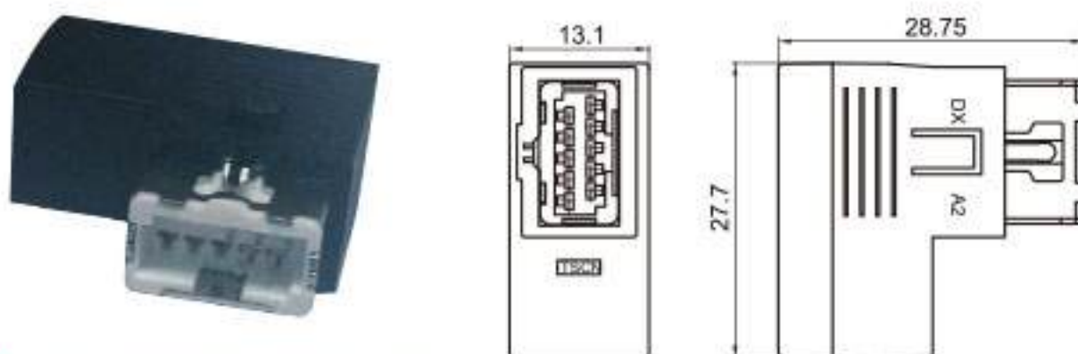
Type: TS3004-10PM-AH-2 Material: PA66 Matching Terminal: TSAM0029 / TSAM0030 / TS 长城 H6
