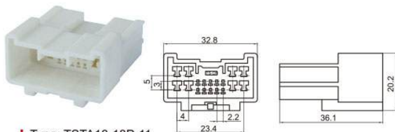
Type: TSTA18-18P-11 Material: PA66 Matching Terminal: TSZ045 / TSZ208
