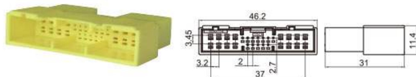
Type: TS30243-28P-11-6 Material: PBT Matching Terminal: TSZ040 / TSZ561A
