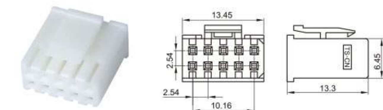
Type: TSCH10-10P-21(10P-24P) Material: PA66 Matching Terminal: TSCH2.5A
