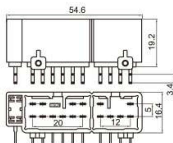
Type: TS1761-16PM-PKB Material: PA66 Matching Terminal: TSPM0002 / TSPM0004 / TSPM0048
