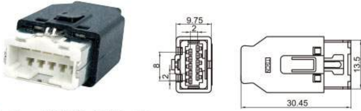
Type: TS3004-10PM-AH Material: PA66 Matching Terminal: TSAM0027 / TSAM0028 / TS 长城 H6
