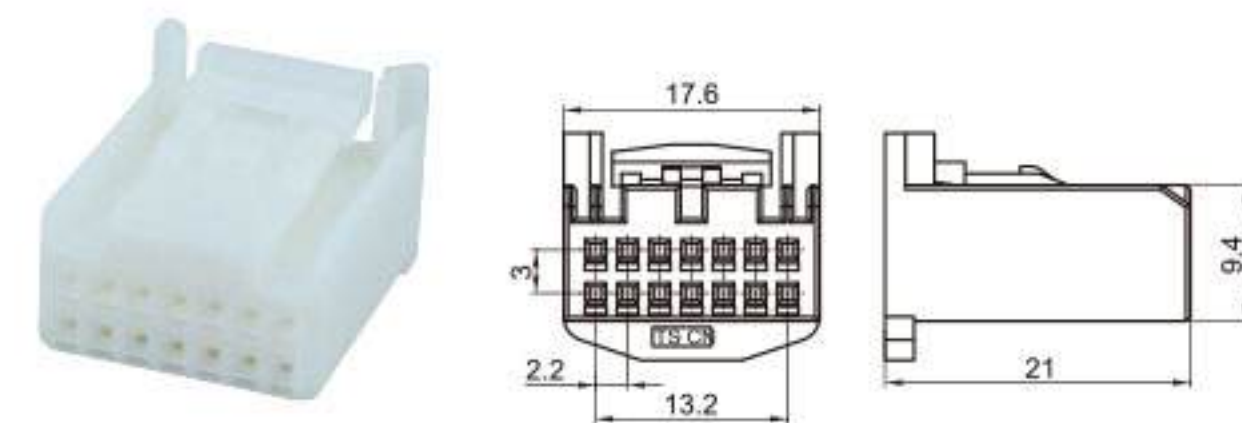
Type: TSTA14-14P-21 Material: PA66 Matching Terminal: TSH143
