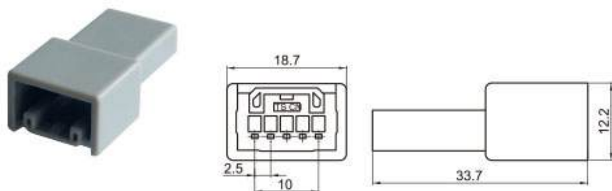
Type: TSTA05-05P-11 Material: PA66 Matching Terminal: TSZ145
