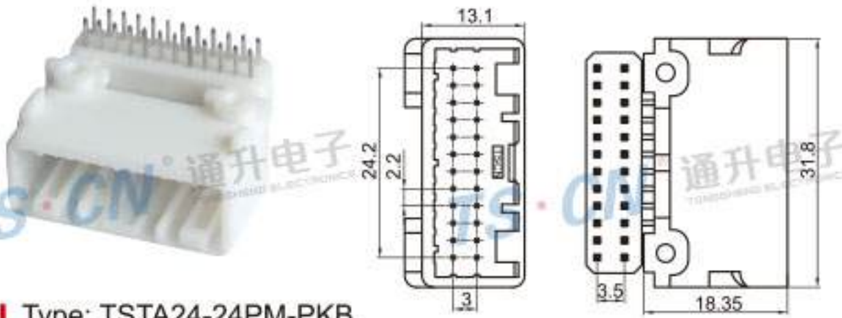
Type: TSTA24-24PM-PKB Material: PA66 Matching Terminal: TSPM0040 / TSPM0041
