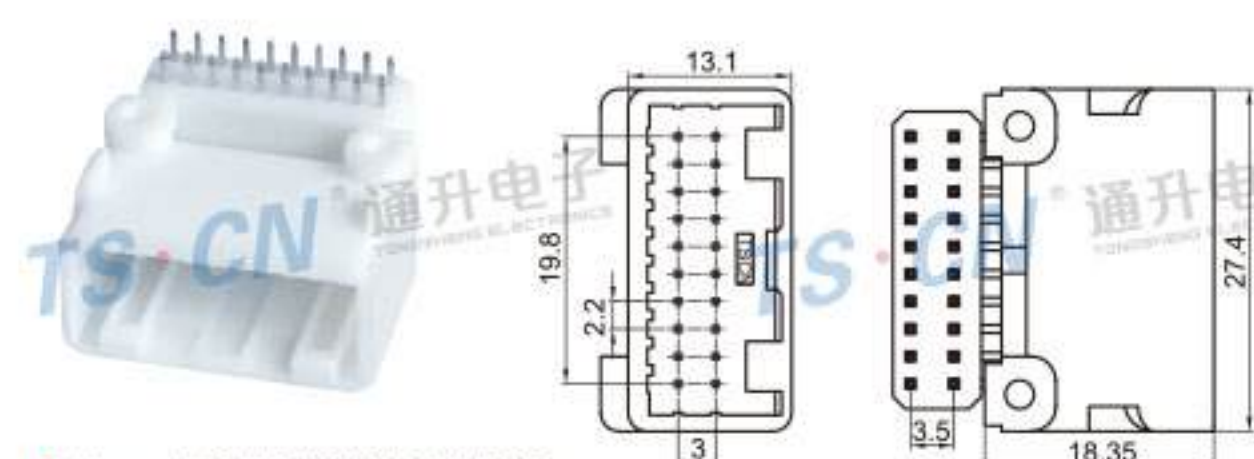
Type: TSTA20-20PM-PKB Material: PA66 Matching Terminal: TSPM0040 / TSPM0041
