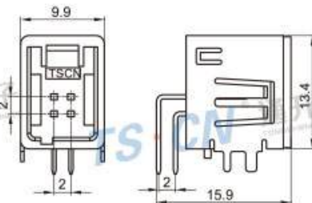
Type: TSMA04-04PM-PKB-4 Material: PPS Matching Terminal: TSPM0029-A / TSPM0031 / TSPM0032
