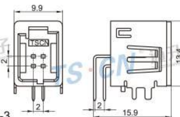
Type: TSMA04-04PM-PKB-3 Material: PPS Matching Terminal: TSPM0029-A / TSPM0031 / TSPM0032
