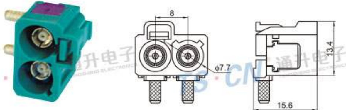
Type: TSVW20-02PF-AT-4 Material: PA66 Matching Terminal: TS 耳机头 -001
