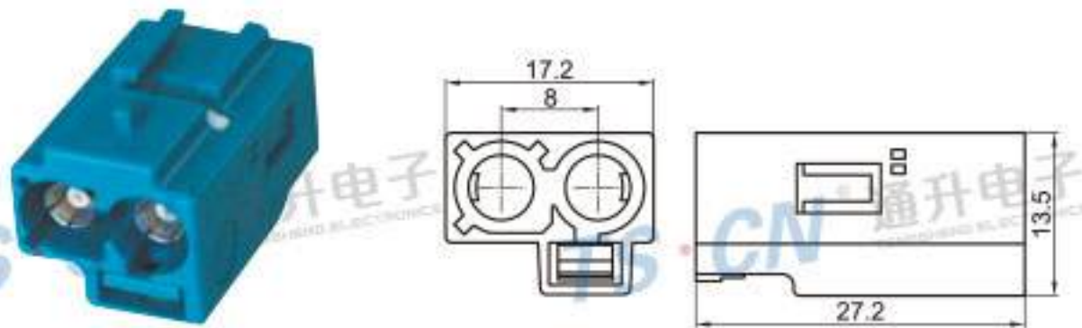
Type: TSVW20-02PF-AT-3 Material: PA66 Matching Terminal: TSTF0025 / TSTF0026
