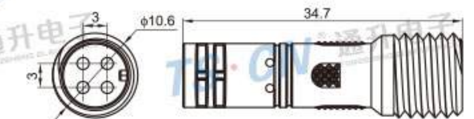
Type: TS 四芯防水公接头 Material: PVC Matching Terminal: TS1.5 圆头
