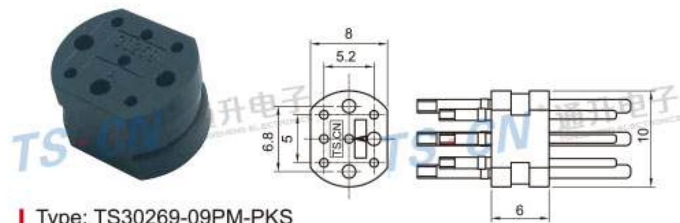
Type: TS30269-09PM-PKS Material: PA66 GF30% Matching Terminal: TS0.9 公针 / TS1.3 公针
