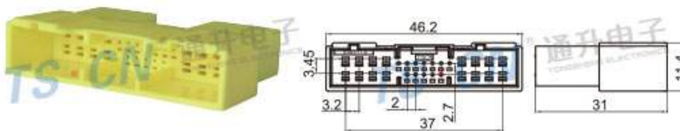
Type: TS30243-28P-11-6 Material: PBT Matching Terminal: TSZ040 / TSZ561A
