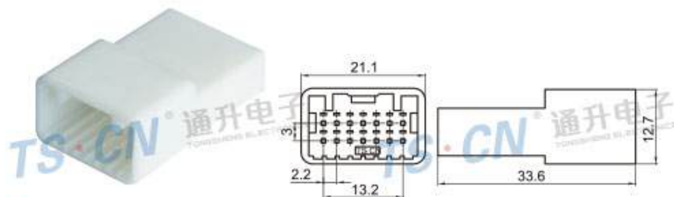
Type: TSTA14-14P-11 Material: PA66 Matching Terminal: TSZ208
