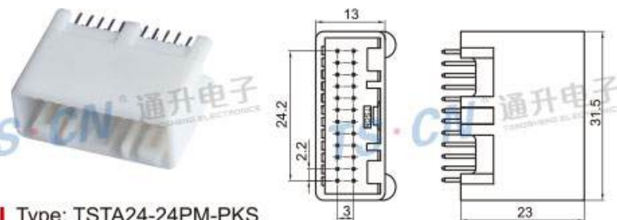
Type: TSTA24-24PM-PKS Material: PA66 Matching Terminal: TSPM0038
