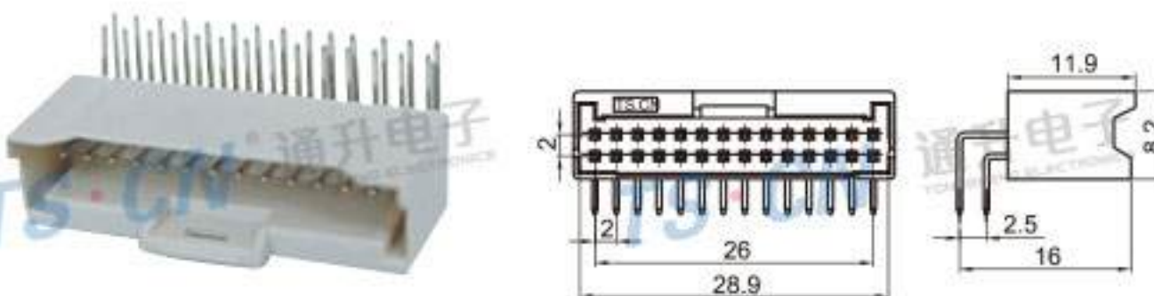
Type: TS30047-28PM-PKB(QRA3) Material: PA66 GF15% Matching Terminal: TSPM0143 / TSPM0144
