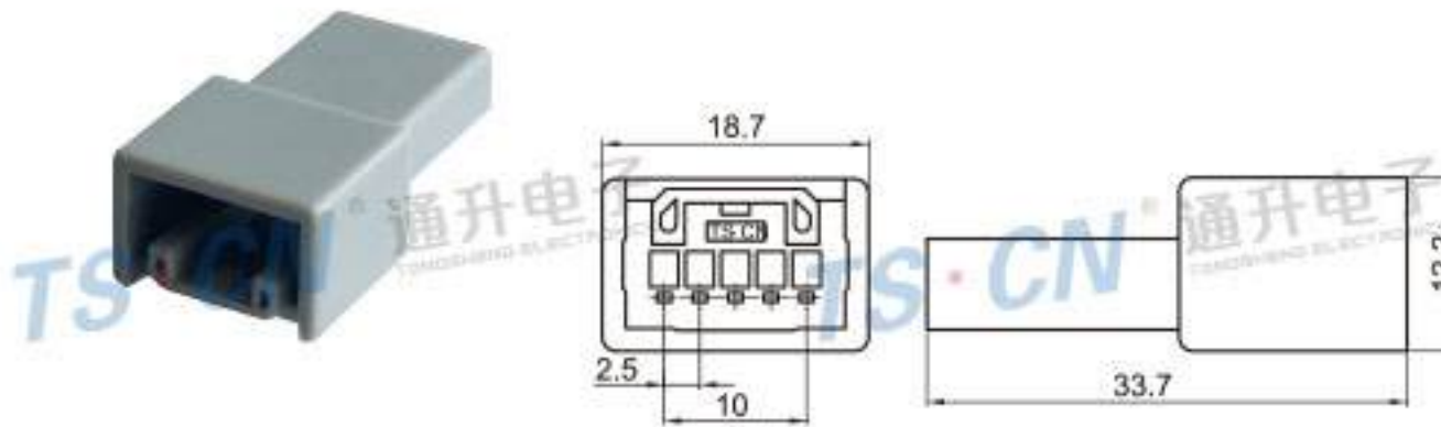
Type: TSTA05-05P-11 Material: PA66 Matching Terminal: TSZ145
