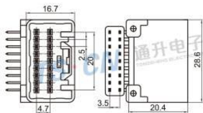
Type: TSMI18-18PM-PKB Material: PA66 Matching Terminal: TSPM0001 / TSPM0003
