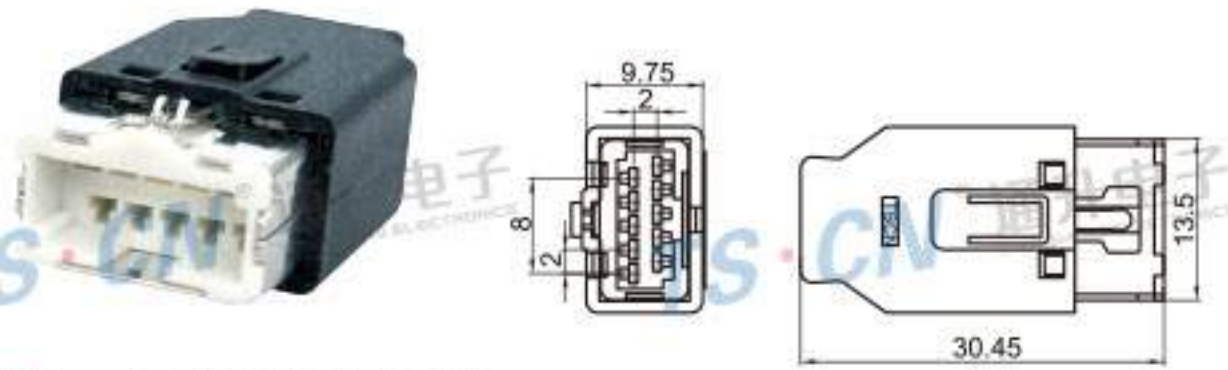
Type: TS3004-10PM-AH Material: PA66 Matching Terminal: TSAM0027 / TSAM0028 / TS 长城 H6
