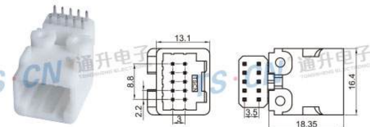
Type: TSTA10-10PM-PKB Material: PA66 Matching Terminal: TSPM0040 / TSPM0041
