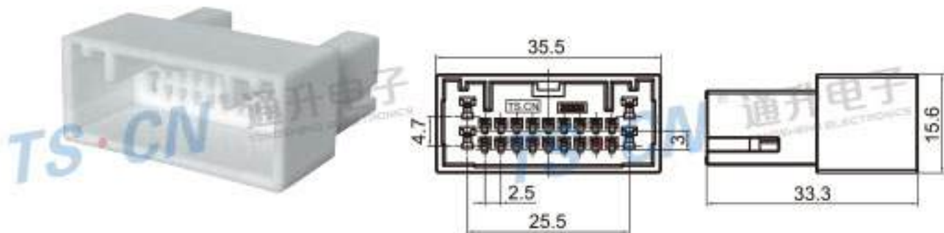
Type: TS30300-22P-11 Material: PBT Matching Terminal: TSZ619 / TSZ618
