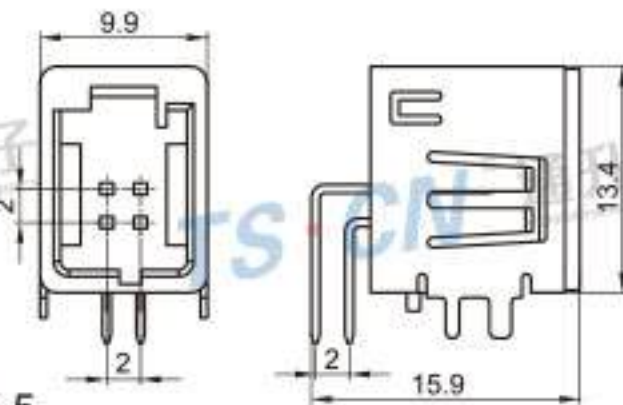
Type: TSMA04-04PM-PKB-5 Material: PPS Matching Terminal: TSPM0029-A / TSPM0031 / TSPM0032
