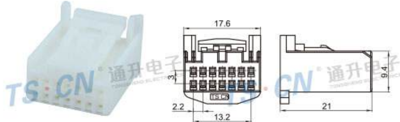
Type: TSTA14-14P-21 Material: PA66 Matching Terminal: TSH143
