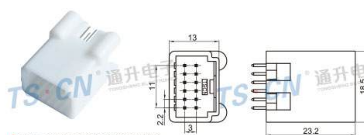
Type: TSTA12-12PM-PKS Material: PA66 Matching Terminal: TSPM0038
