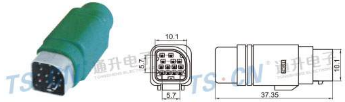
Type: TSALP13-13PM-AH Material: PA66 Matching Terminal: TSAM0016 / TSAM0015 / TS0079
