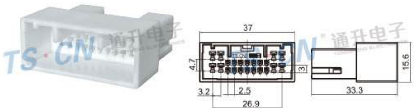
Type: TS30300-22P-11-1 Material: PBT Matching Terminal: TSZ619 / TSZ618
