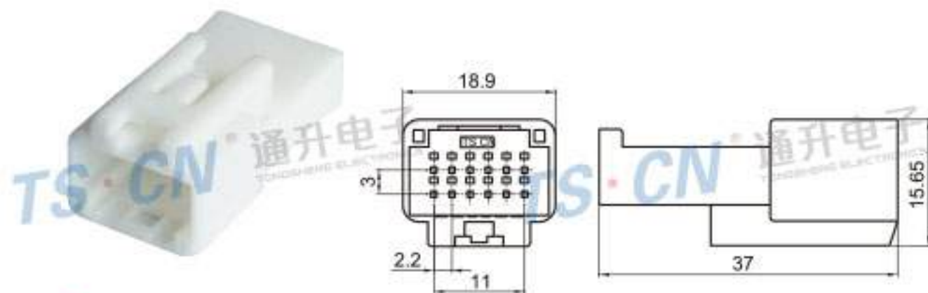
Type: TSTA12-12P-11 Material: PA66 Matching Terminal: TSZ208
