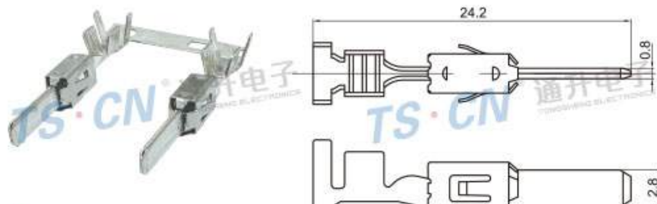
Type: TSZ625 Material: Phos.bronze
