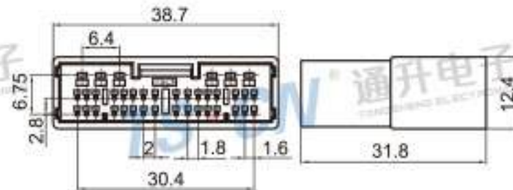
Type: TS30101-38P-11 Material: PA66 Matching Terminal: TSZ562 / TSZ556
