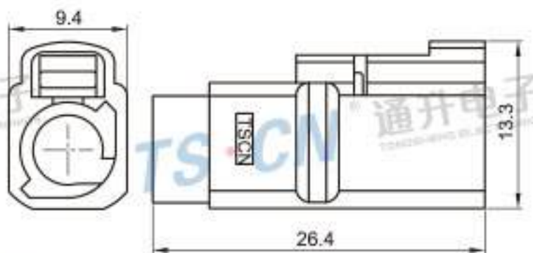
Type: TSVW20-01PF-AT-LG Material: PA66 GF30% Matching Terminal: TSTF0025 / TSTF0026
