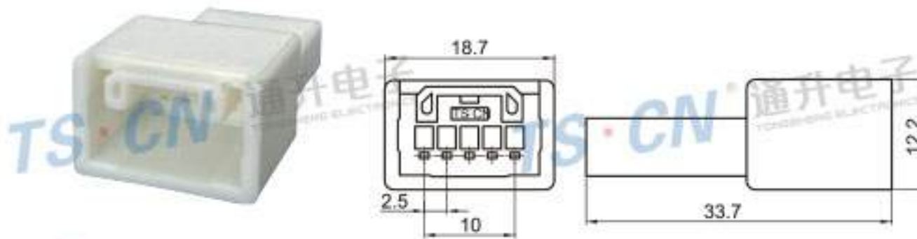
Type: TSTA05-05P-11-1 Material: PA66 Matching Terminal: TSZ145
