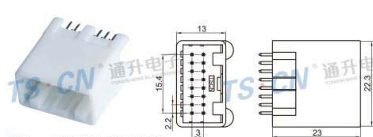
Type: TSTA16-16PM-PKS Material: PA66 Matching Terminal: TSPM0038
