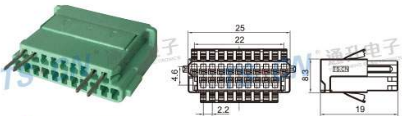
Type: TS30304-86P-11-C Material: PBT Matching Terminal: TSZ618
