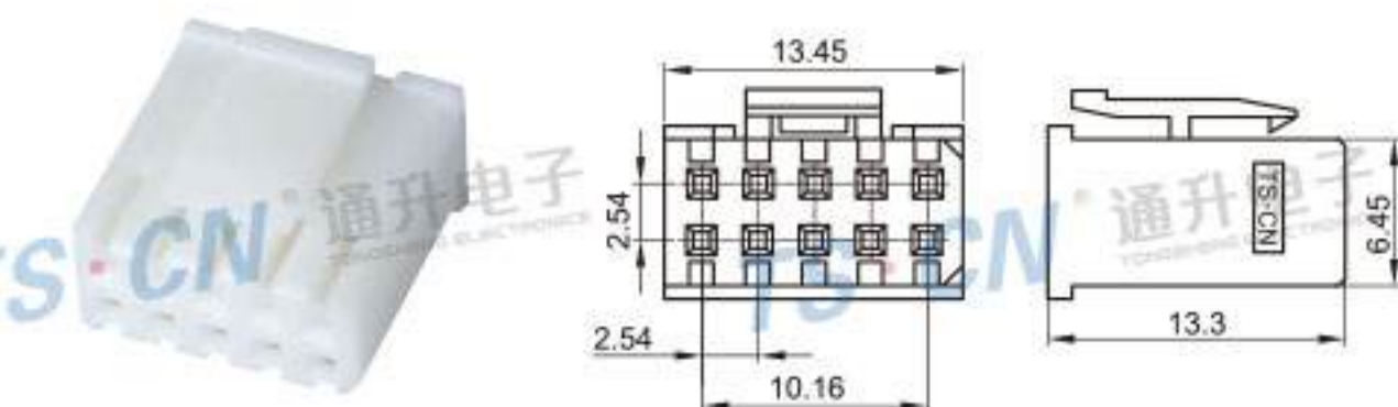
Type: TSCH10-10P-21(10P-24P) Material: PA66 Matching Terminal: TSCH2.5A
