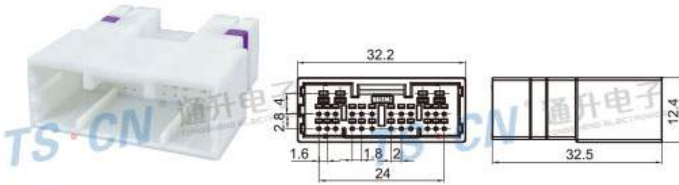
Type: TS30101-28P-11-5 Material: PA66 Matching Terminal: TSZ562 / TSZ615
