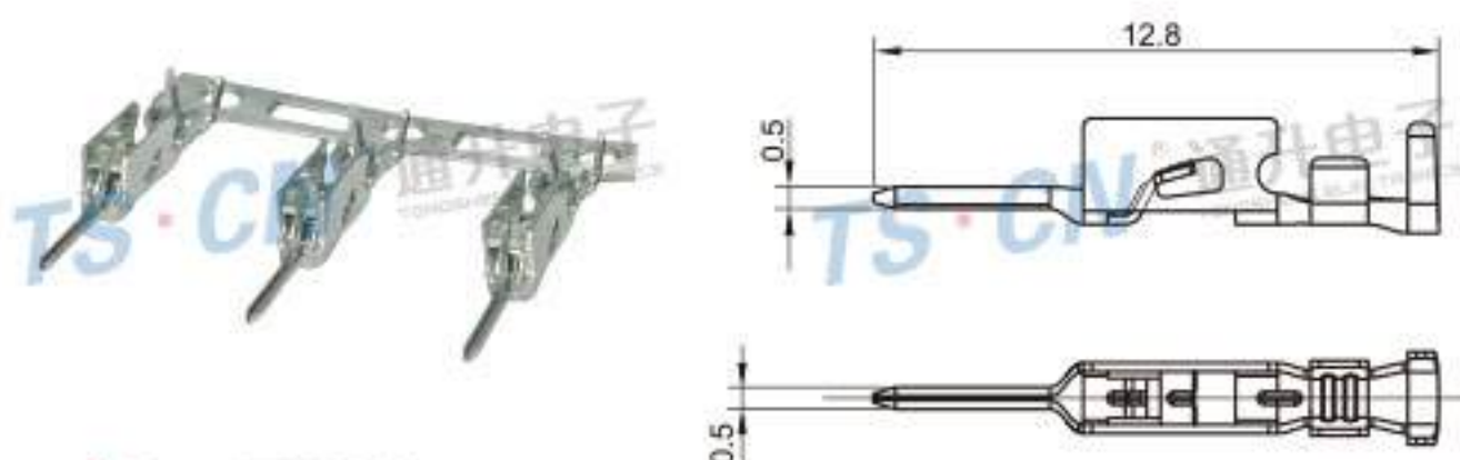
Type: TSZ622 Material: Phos.bronze
