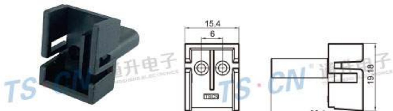
Type: TS30353-02P-11 Material: PBT Matching Terminal: TSZ620
