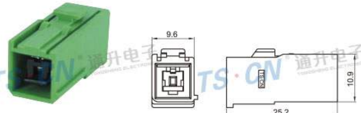
Type: TSFIAT20-01PF-AT-2 Material: PA66 Matching Terminal: TSTF0014-A/TSTF0015
