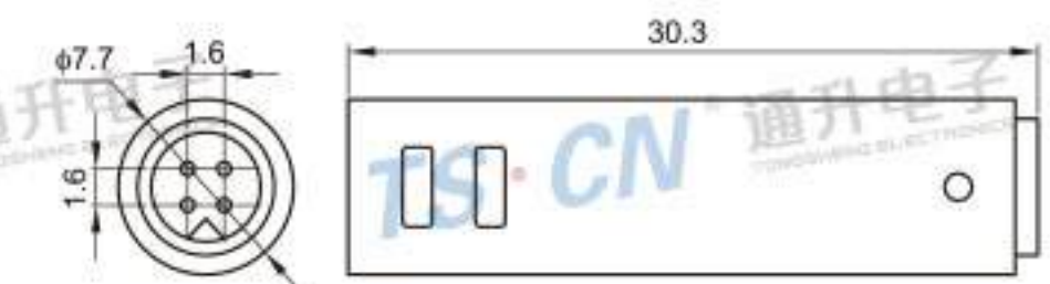
Type: TSBMP4 公 Material: PVC Matching Terminal: TSMB4P-M
