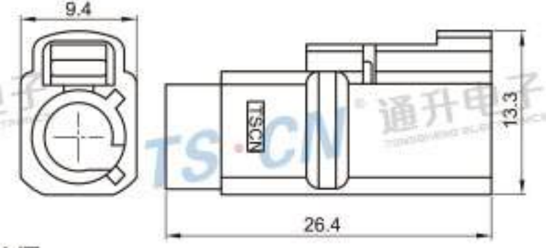
Type: TSVW20-01PF-AT-VT Material: PA66 GF30% Matching Terminal: TSTF0025 / TSTF0026
