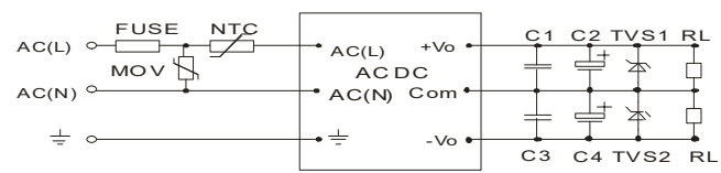
图2: 正负双路系列典型应用电路
