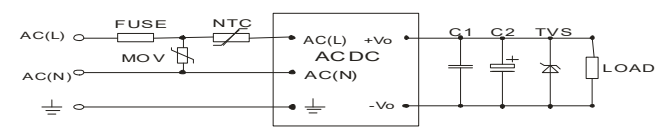
图1: 单路系列典型应用电路
