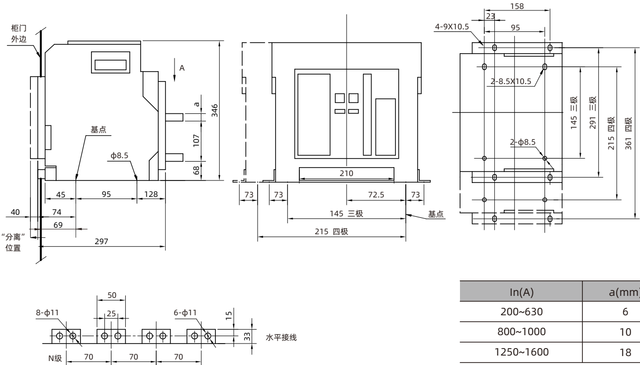
□ W3-1600/3P、4P抽屉式安装尺寸
