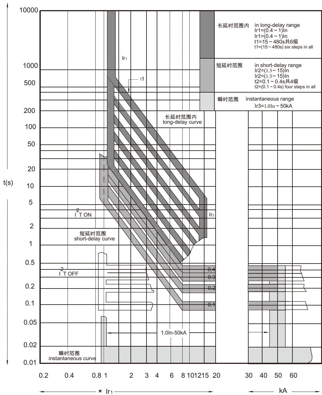
智能控制器时间/电流特性曲线
