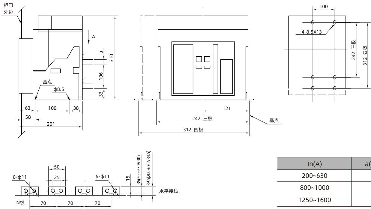
□ W3-1600/3P、4P固定式安装尺寸
